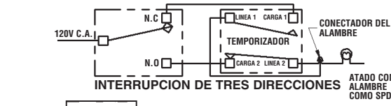
INTERRUPCION DE TRES DIRECCIONES
